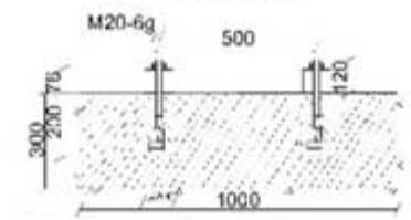
Б-Б (1:10)
