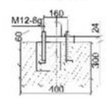
В-В (1:10)
